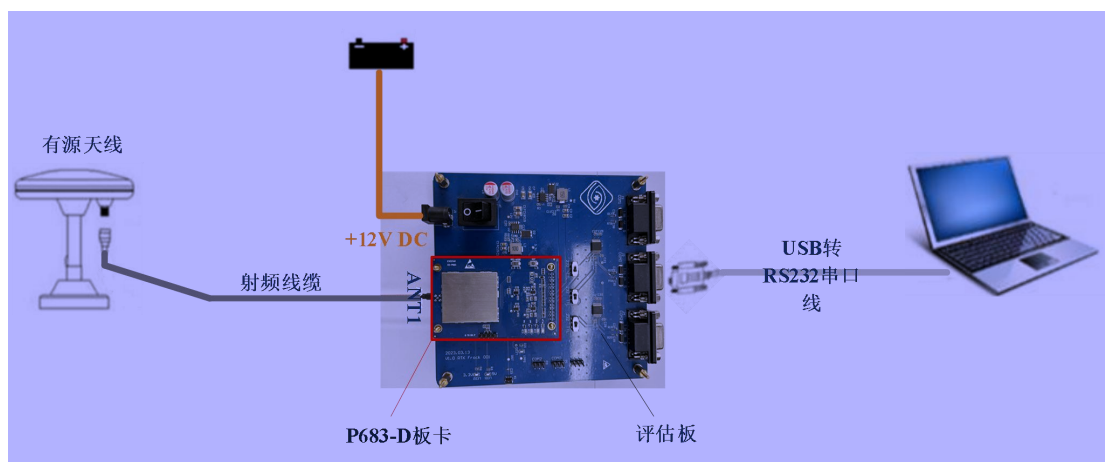
图 4-1 P683-D 连接示意图
