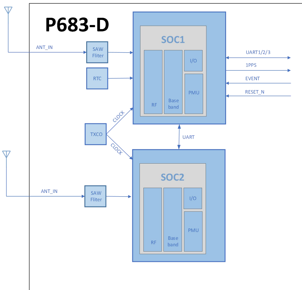
图 1-2 P683-D 系统框图
