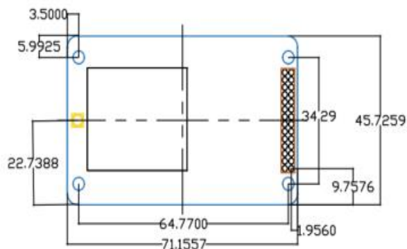
图 2-1 机械结构框图
