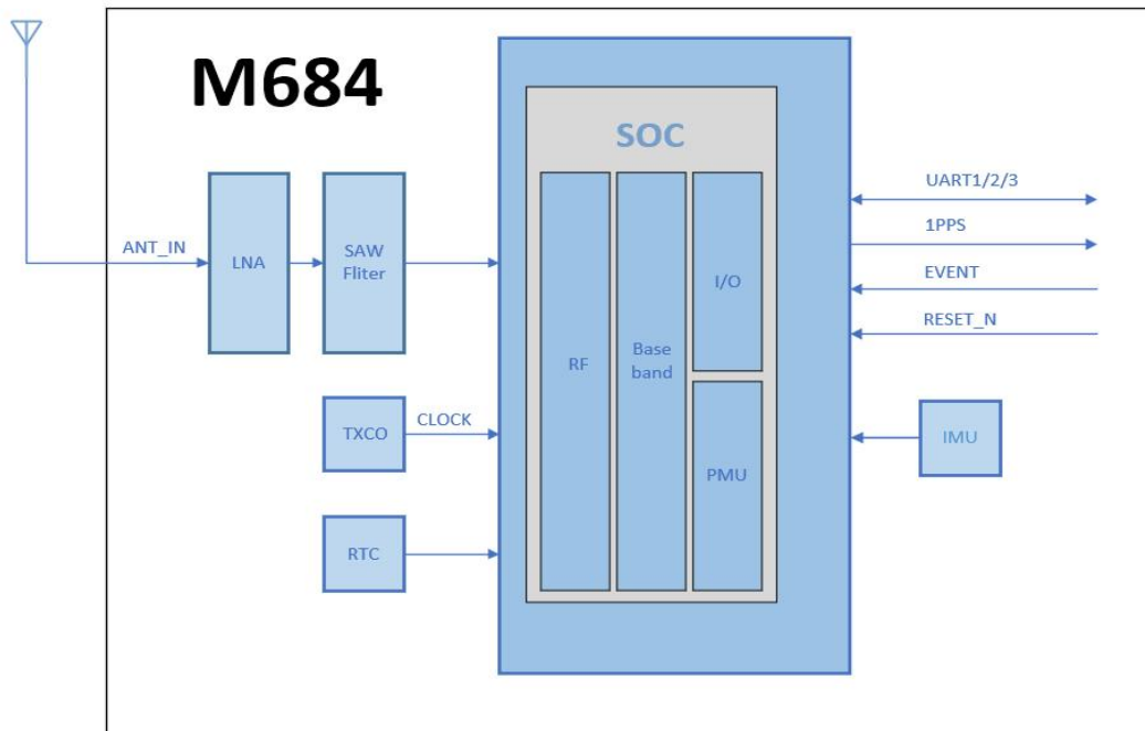
图 1-2 M684 系统框图
