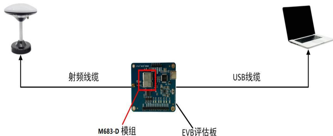
图 4-1 连接示意图
