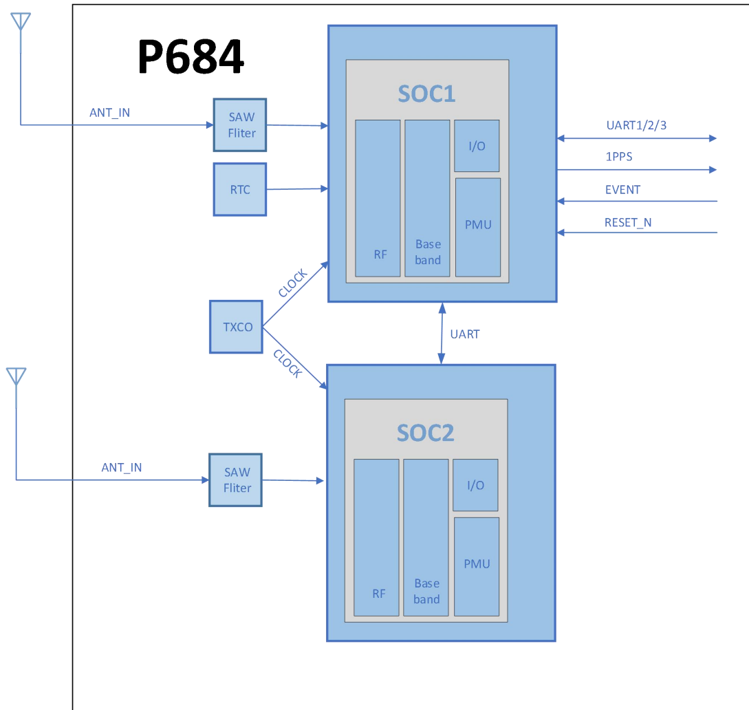
图 1-2 P684 系统框图
