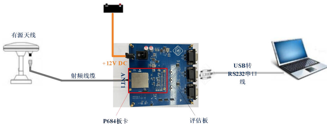
图 4-1 P684 连接示意图
