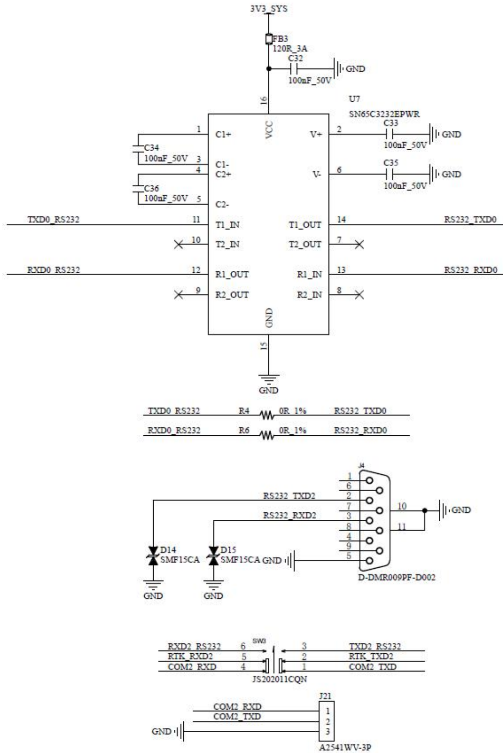
图 3-2 P684 接口参考电路设计
