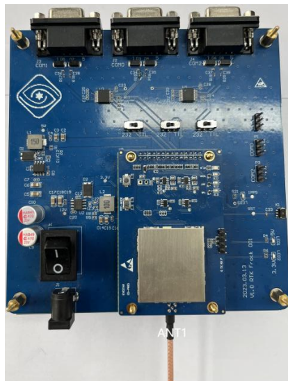
图 4-2 连接天线
