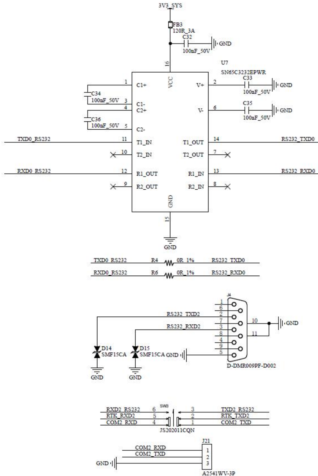
图 3-2 P684-D 接口参考电路设计
