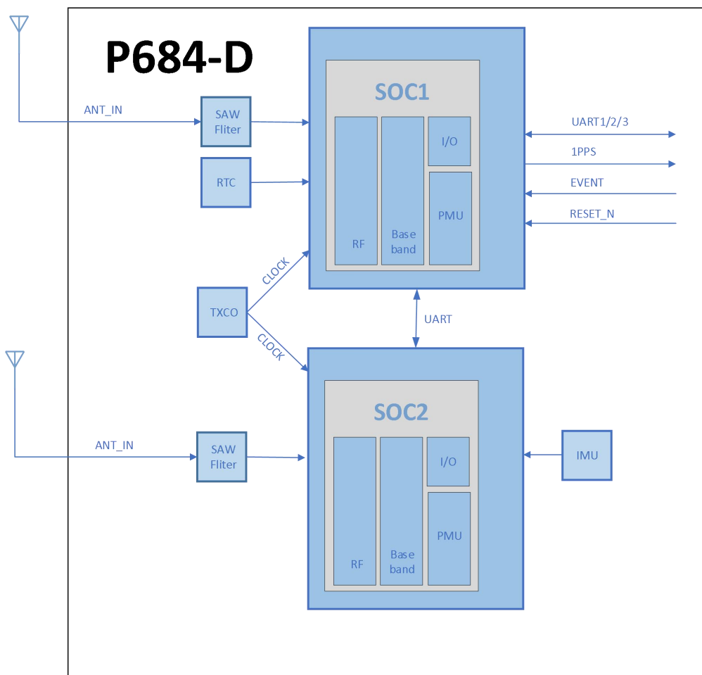
图 1-2 P684-D 系统框图
