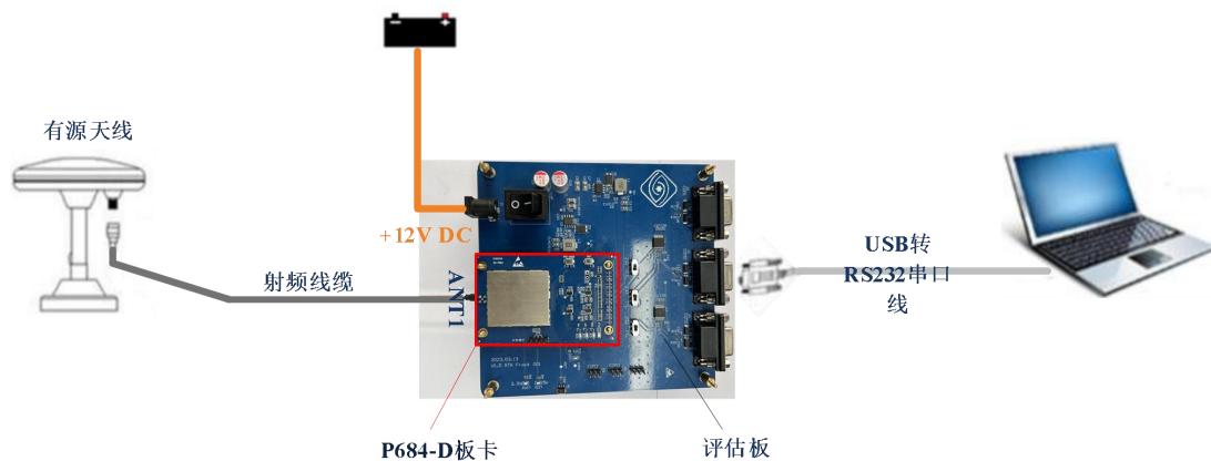
图 4-1 P684-D 连接示意图
