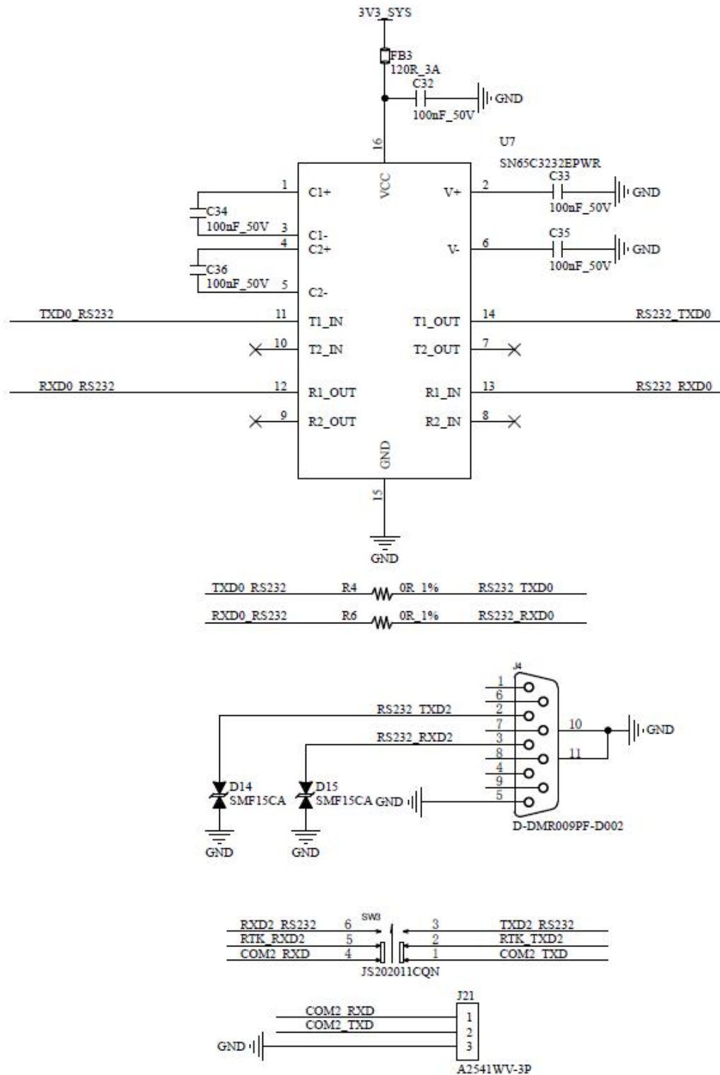
图 3-2 P683 接口参考电路设计
