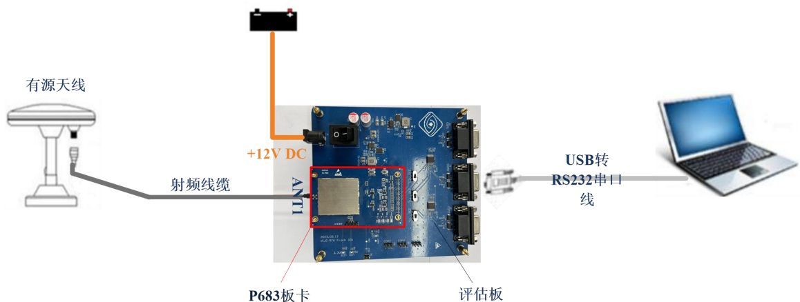
图 4-1 P683 连接示意图
