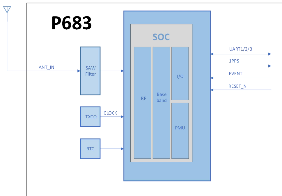
图 1-2 P683 系统框图
