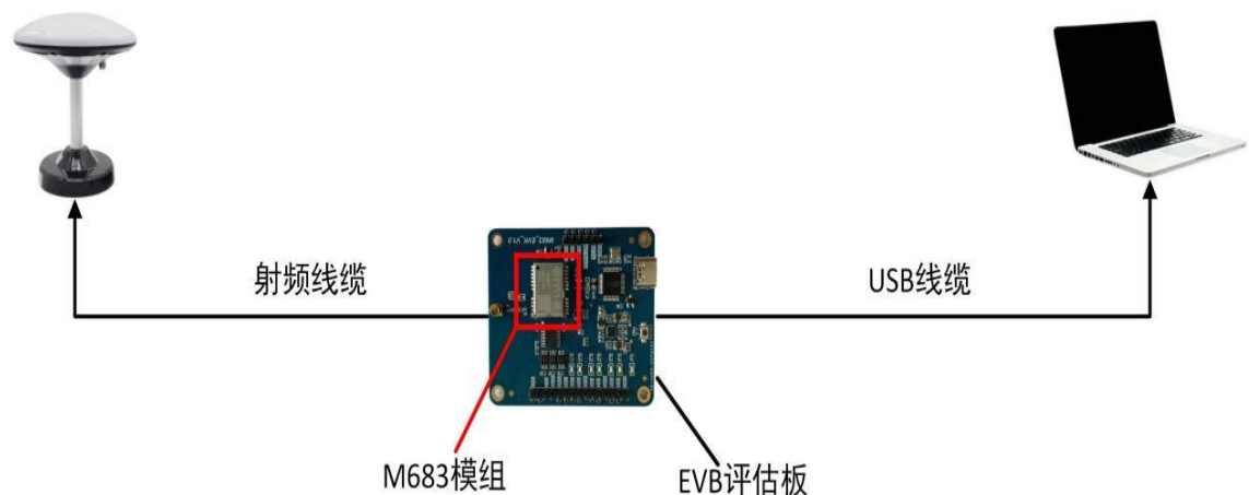
图 4-1 连接示意图
